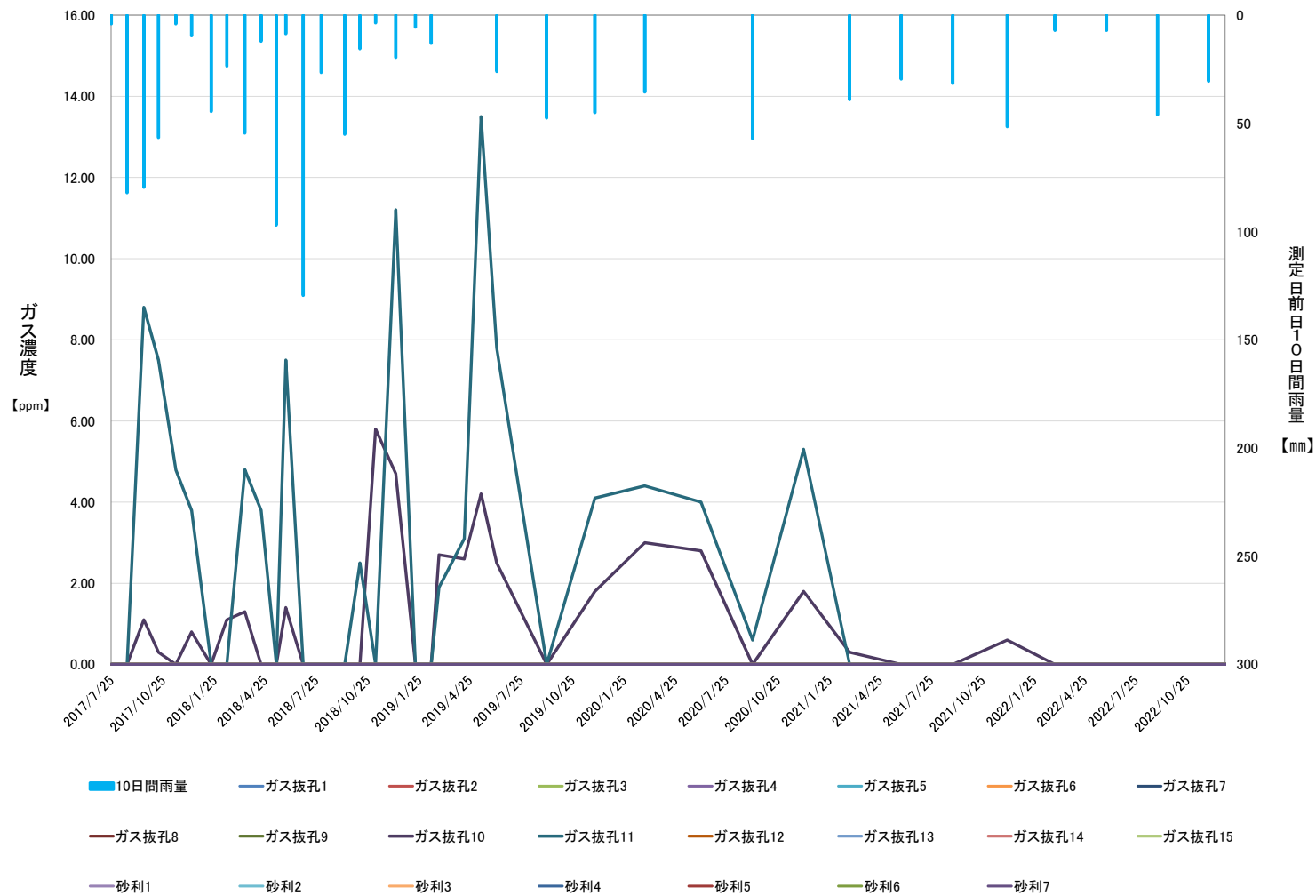
各観測地点の硫化水素ガス濃度経年変化
